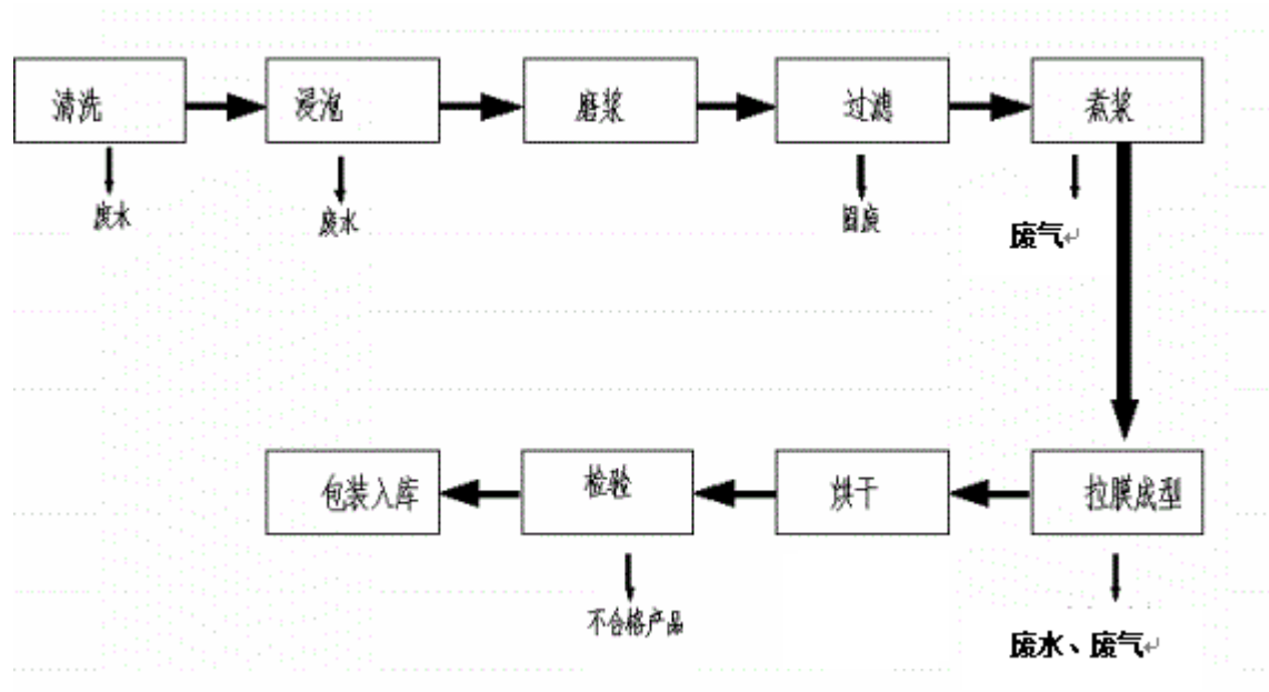
图 5-2 本项目腐竹生产工艺流程及产排污节点图
