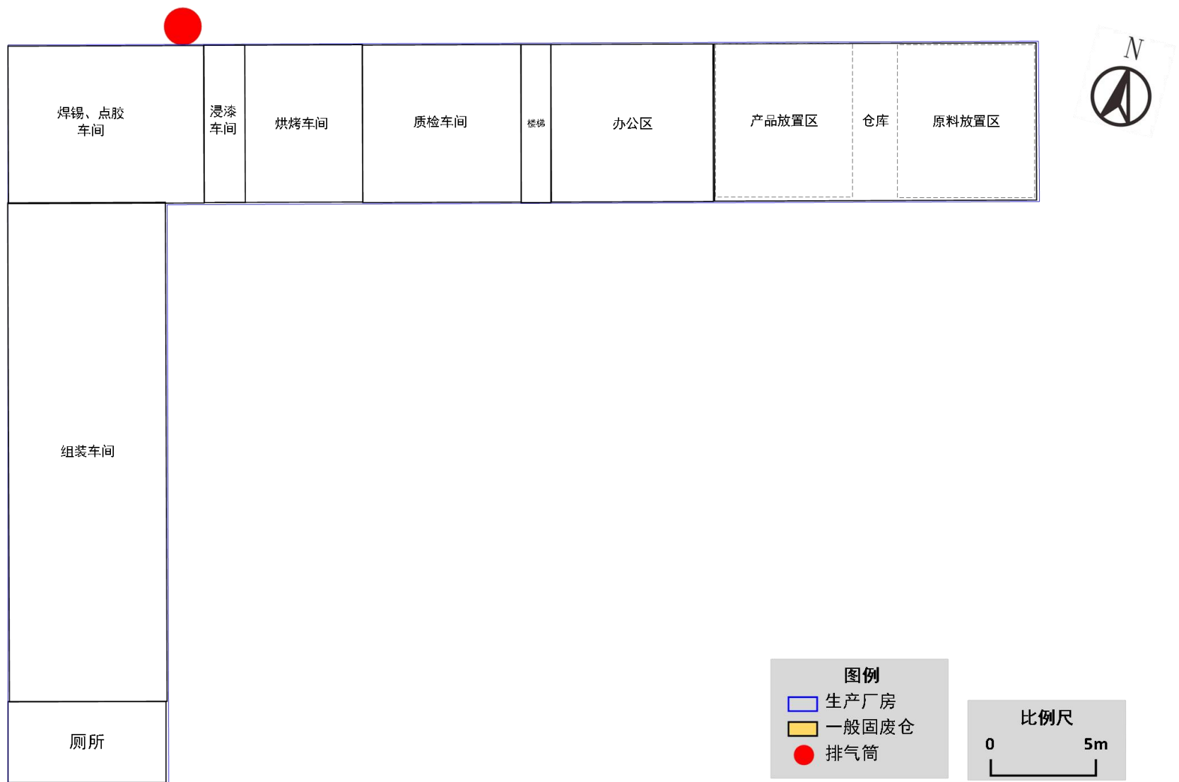
附图 4-1 1 层平面布置图
