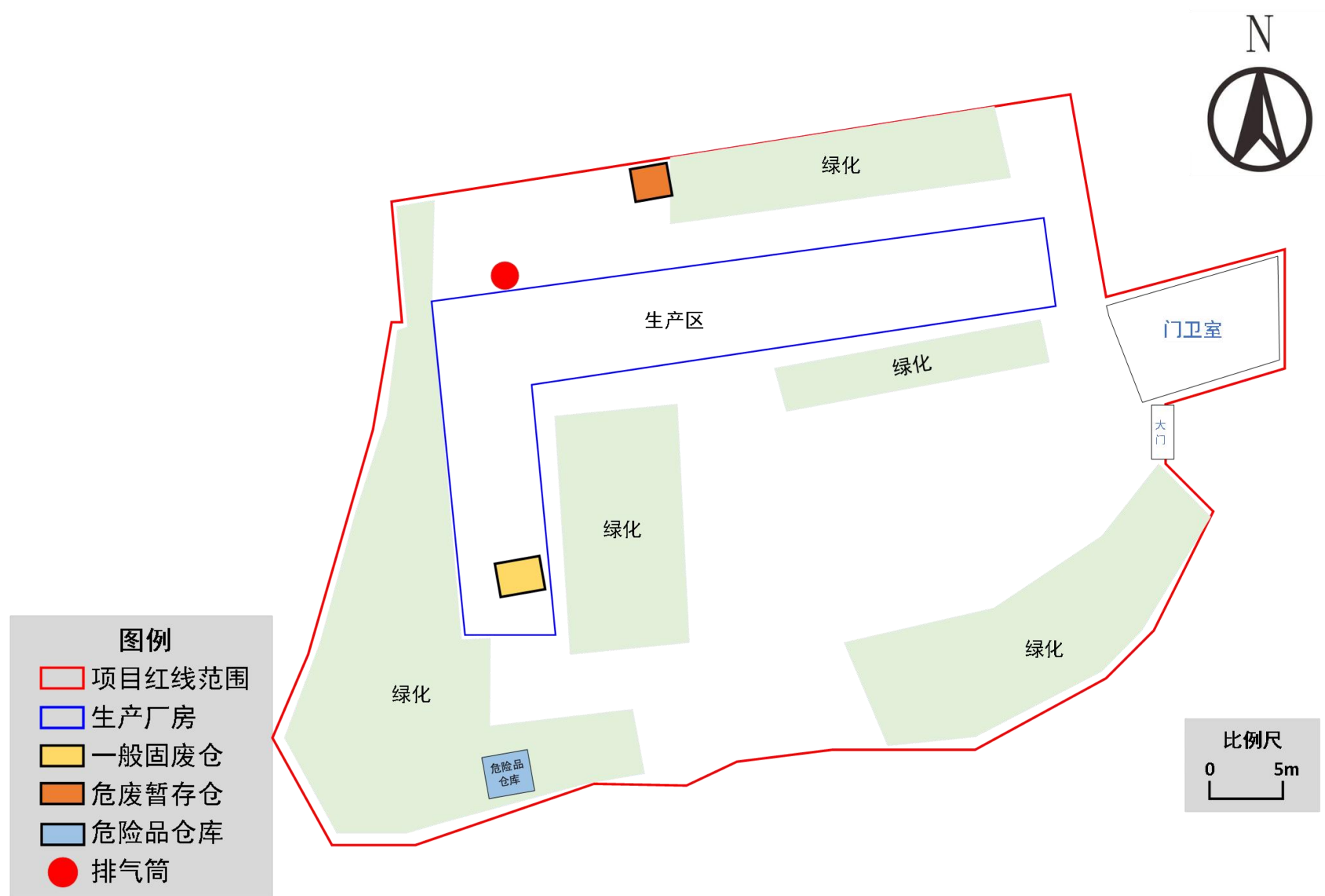
附图 4-3 项目总平面布置图
