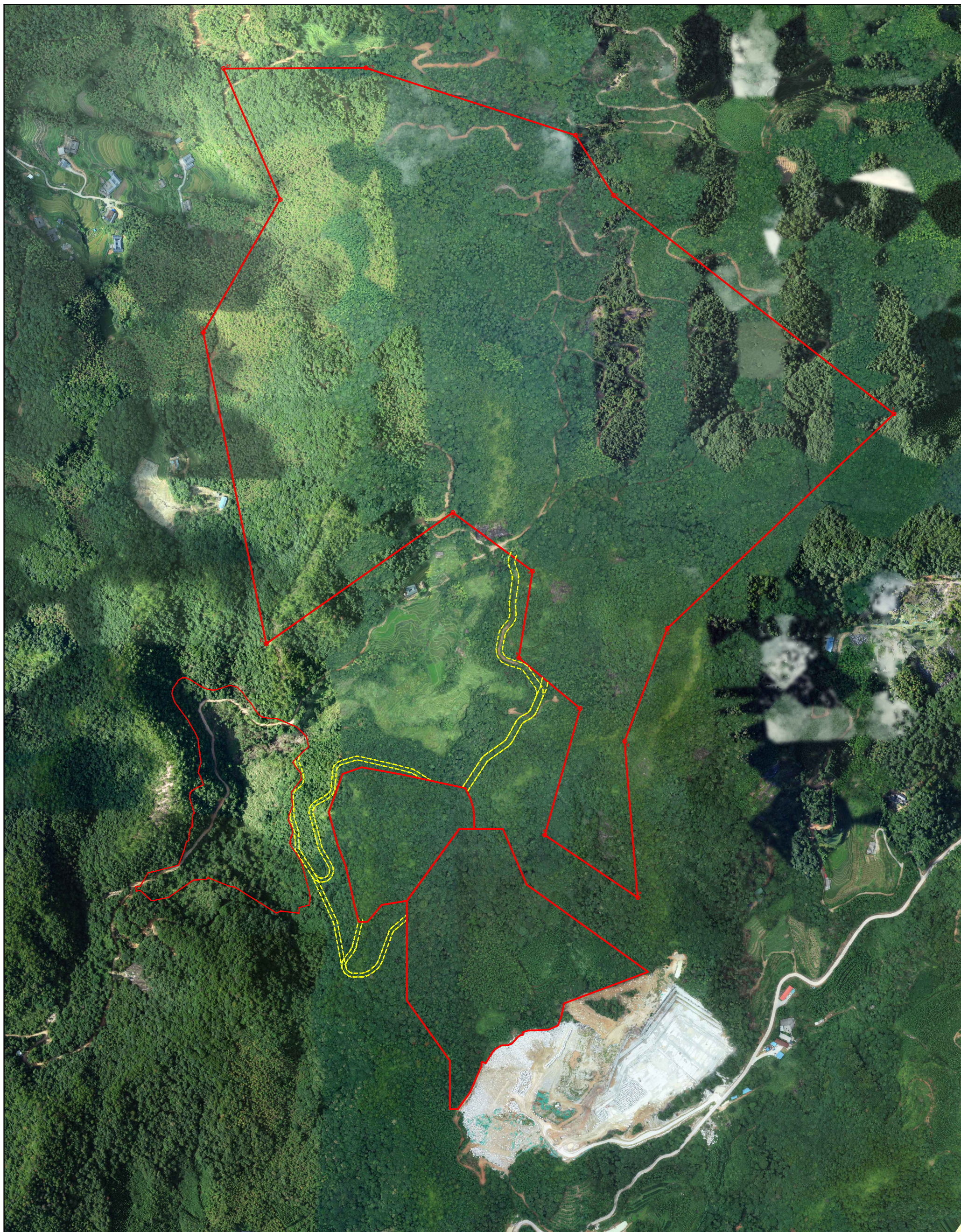
仁居镇木溪矿区拟征地范围及影像图
