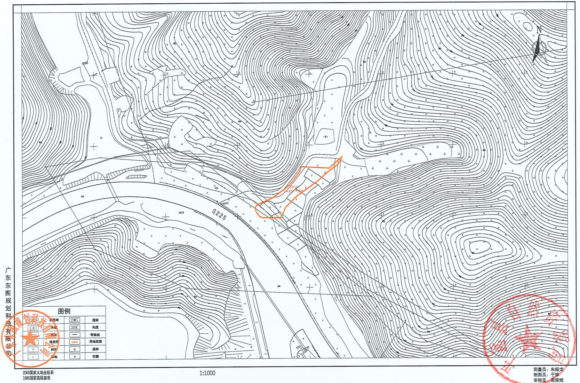
平远县2024年度第二十三批次城镇建设用地勘测定界图（四）
