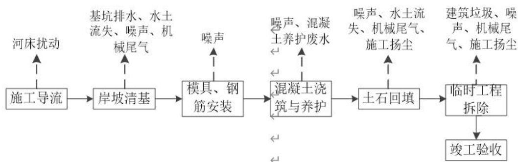
图 2-2 施工工艺流程及产污位置图
