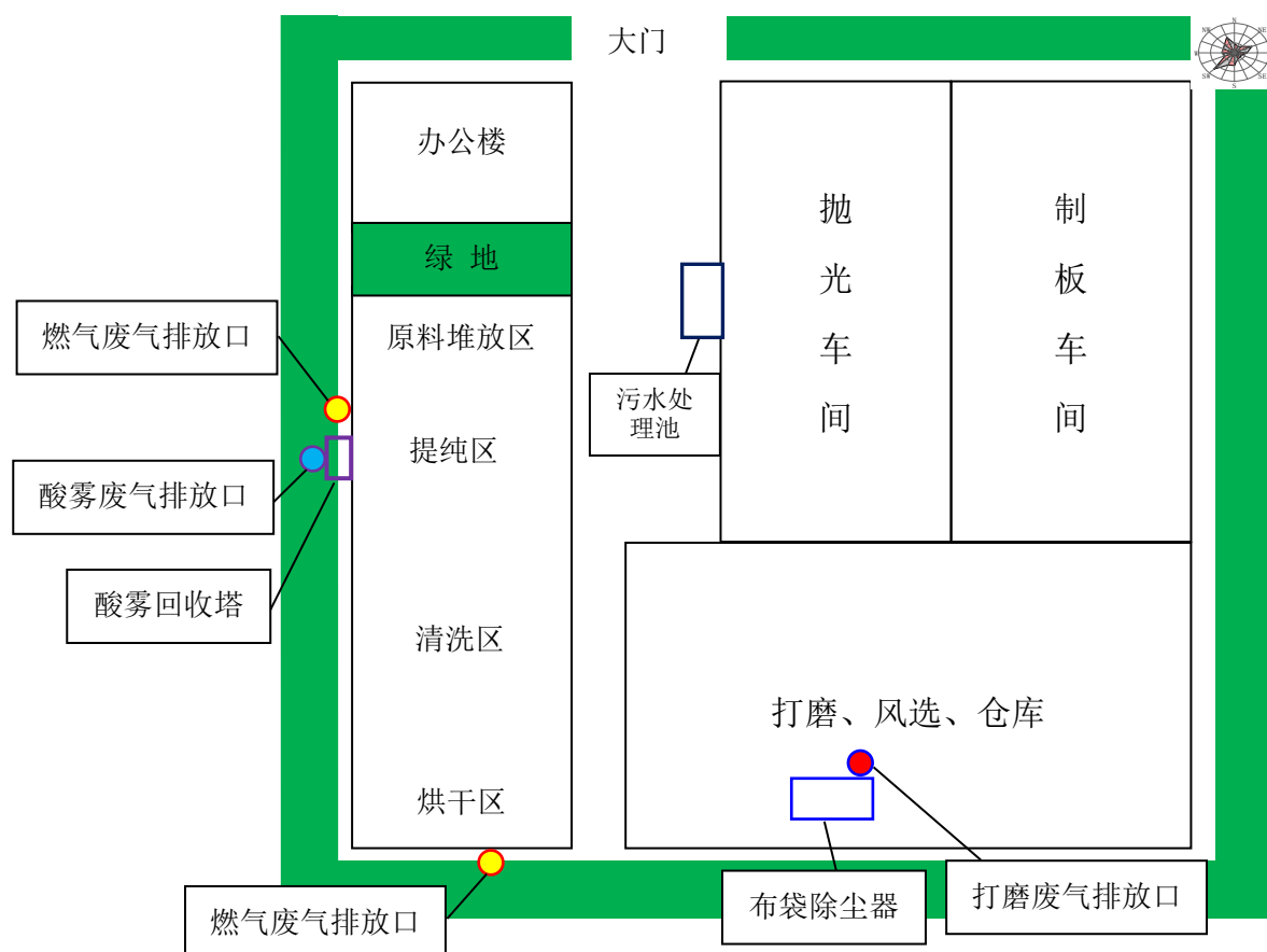
附图 3 车间平面布置图
