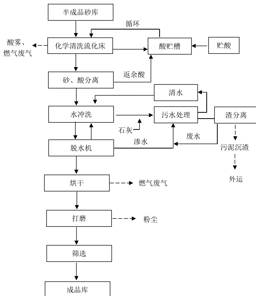
图 5-1 高纯砂化学提纯流程图
