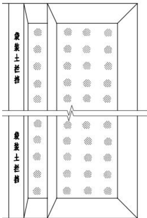
图 5-1 表土剥离堆放区设计示意图
