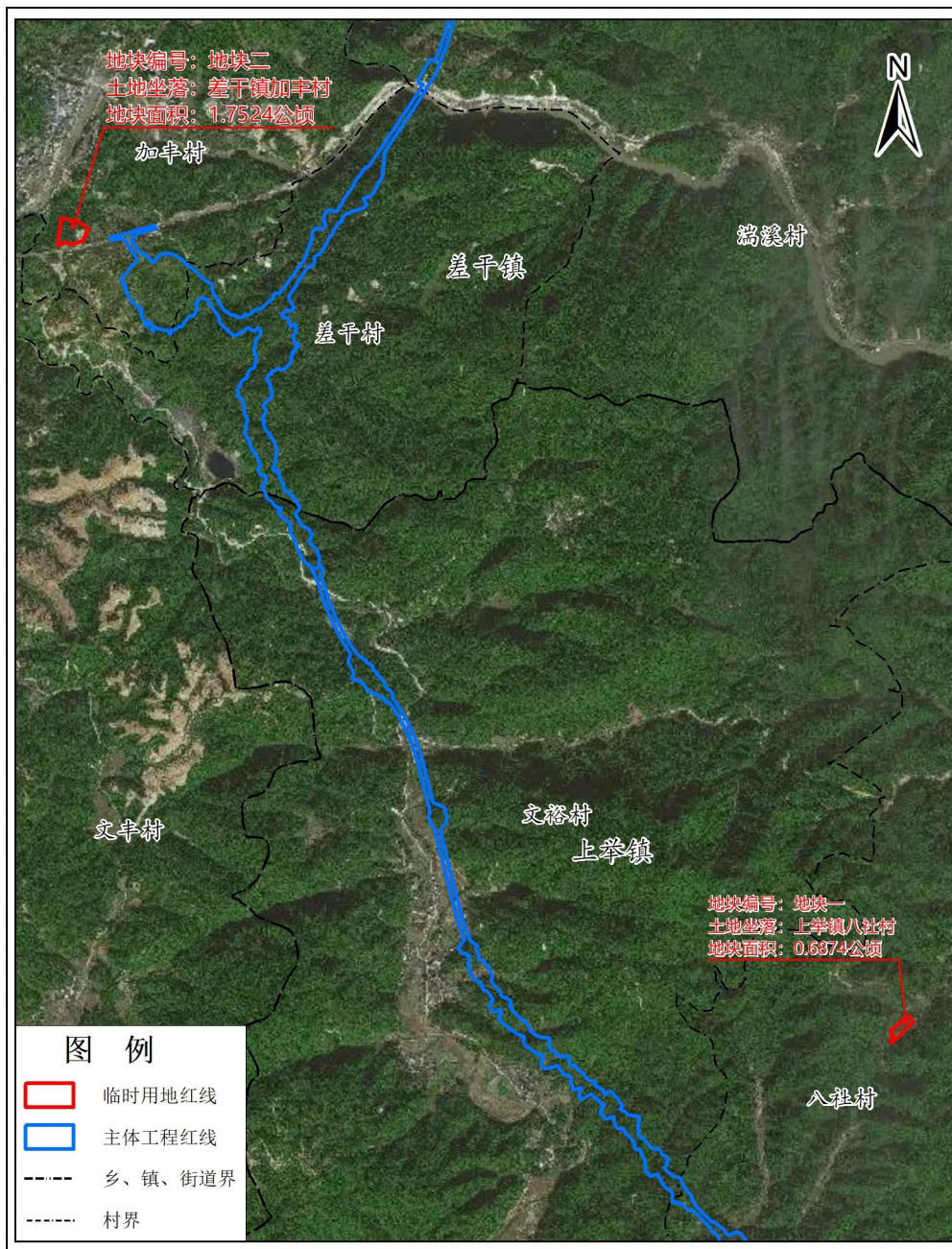
图3-1 临时用地与主体工程套合图
